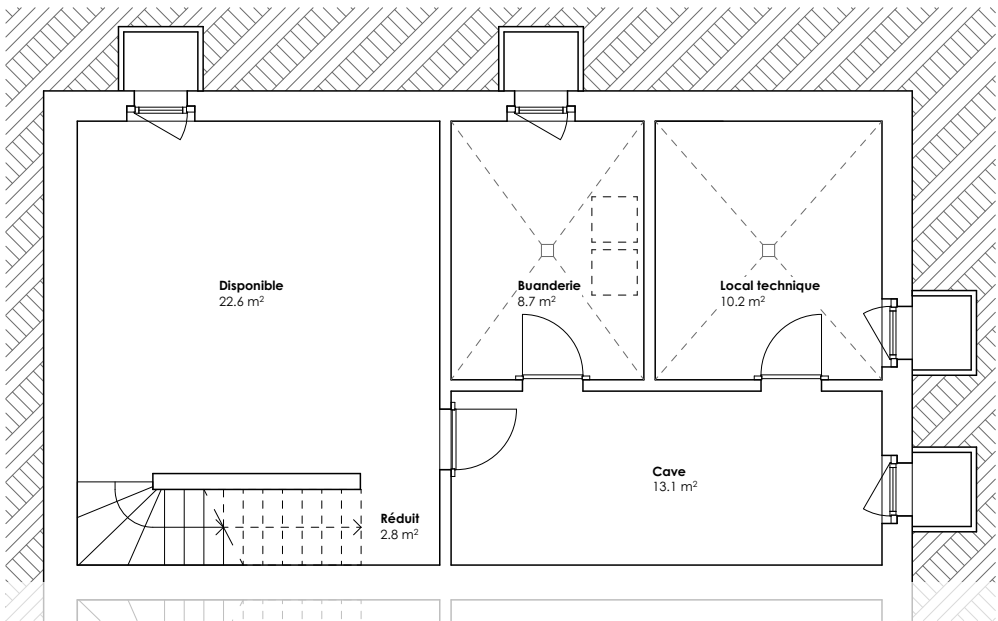
Sous-sol 1/100 e
