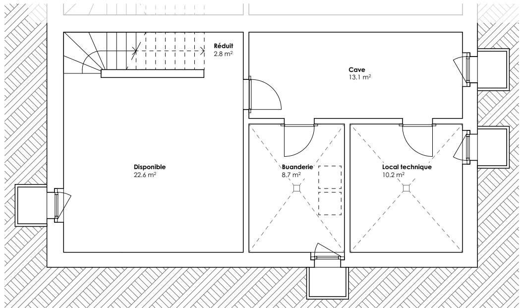
Sous-sol 1/100 e
