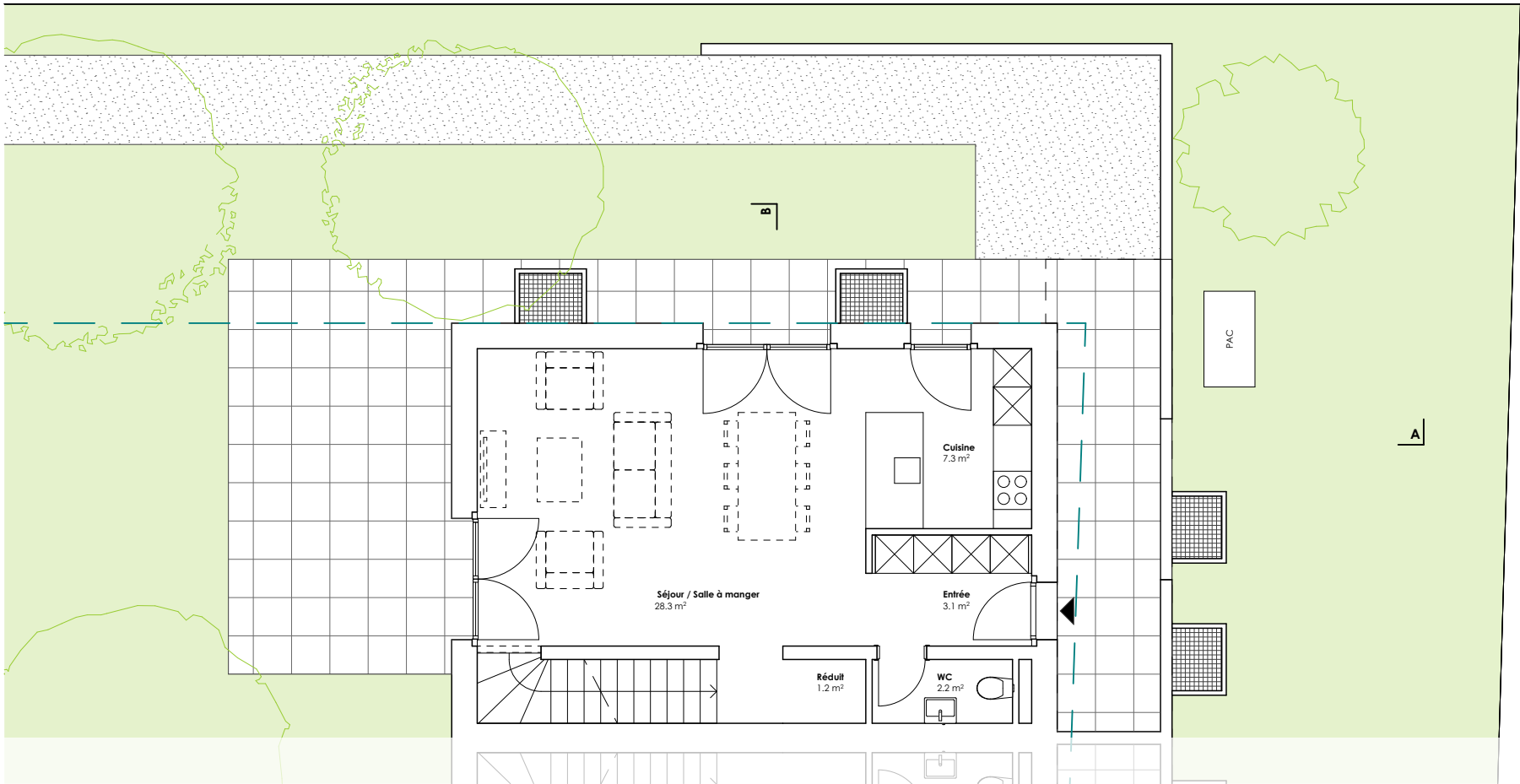
Rez-de-chaussée 1/100 e
