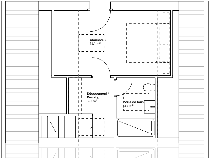
Combles 1/100 e
