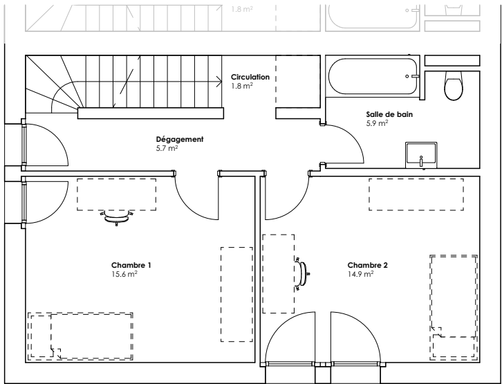
Etage 1/100 e
