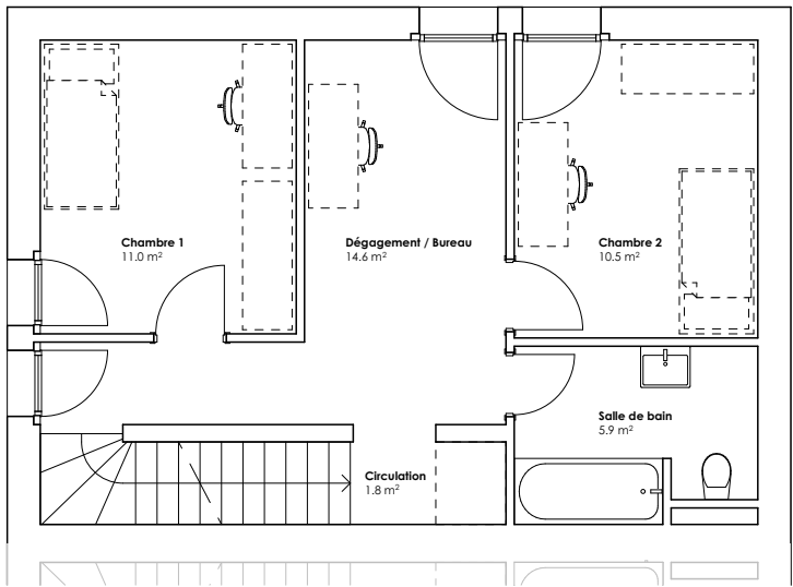
Etage 1/100 e
