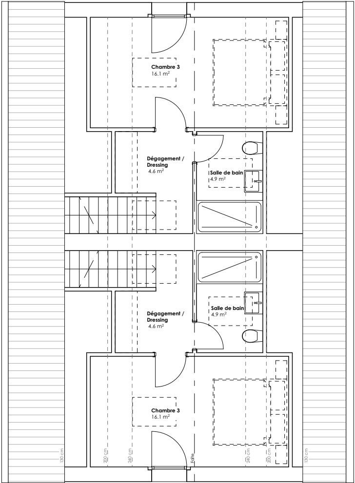
Variante n°1
